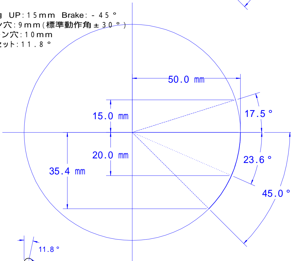
エルロンリンケージ設定図
