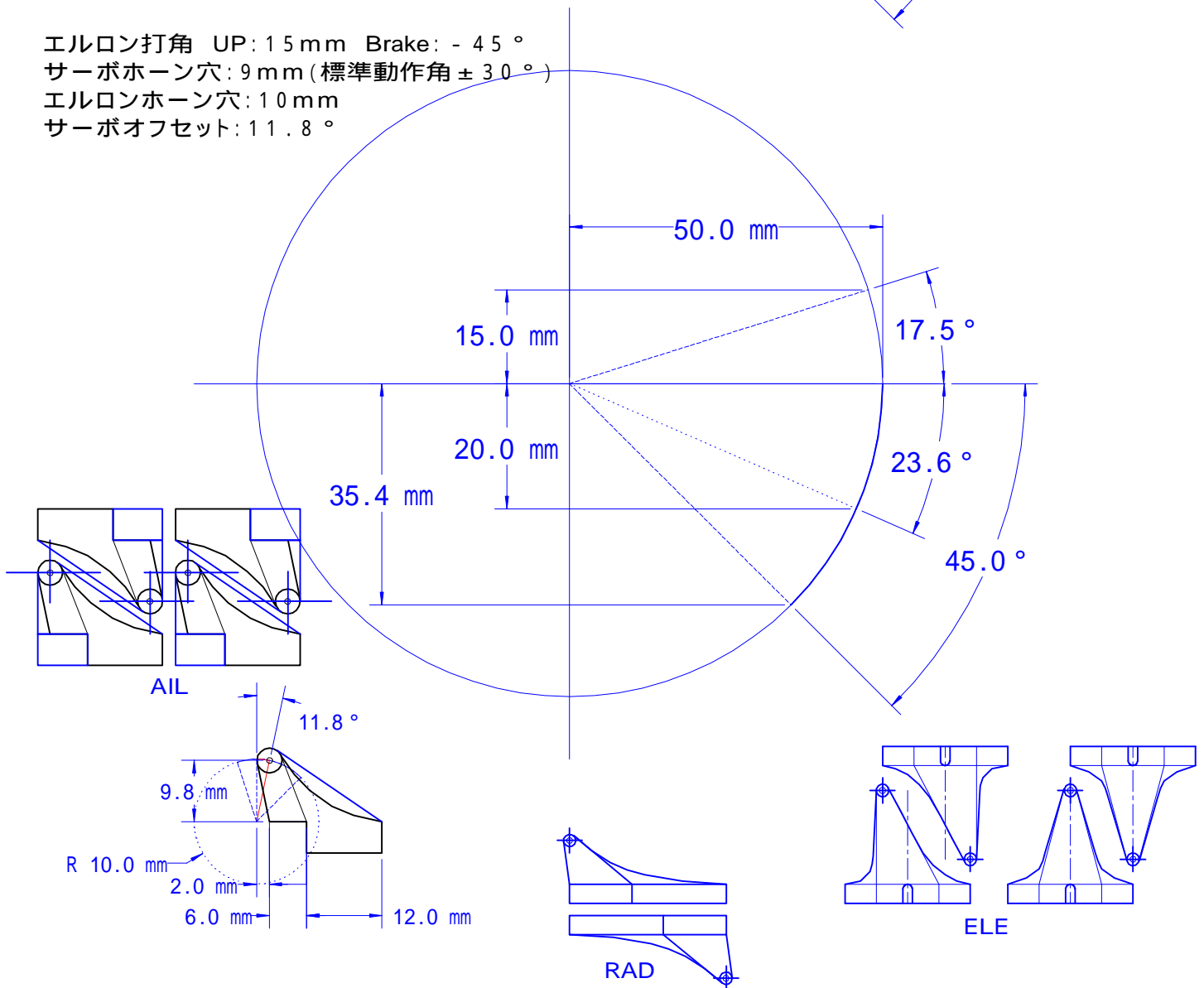
エルロンリンケージ設定図
